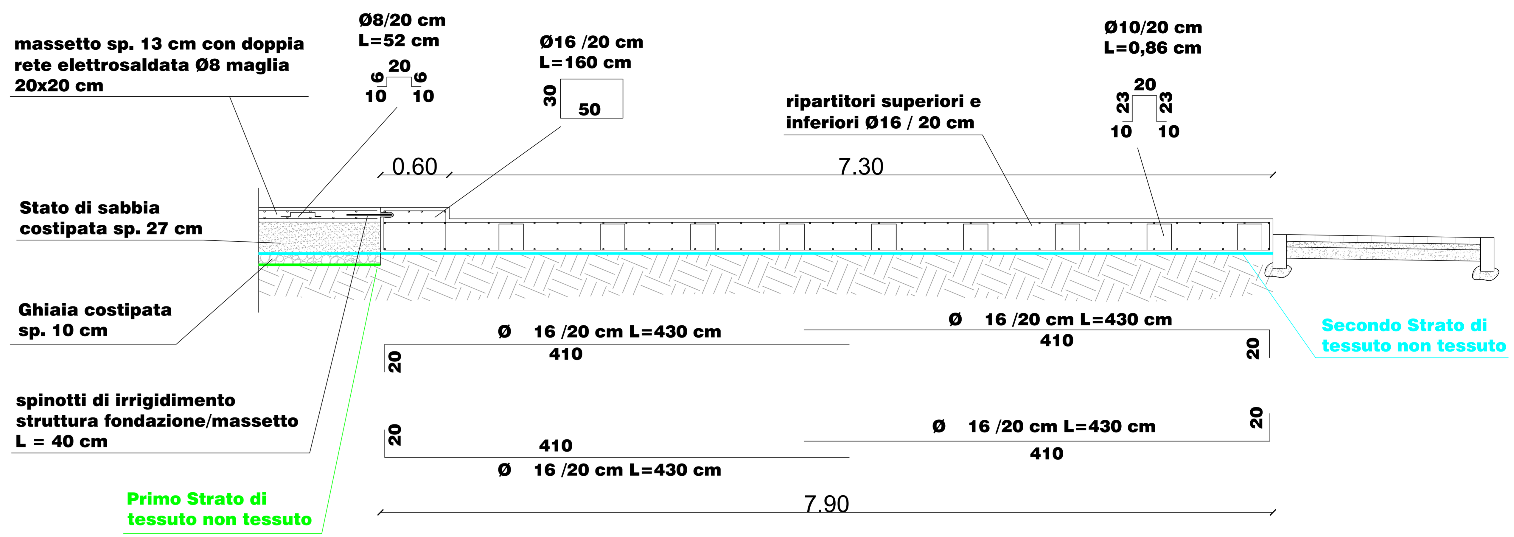
SEZIONE D-D
